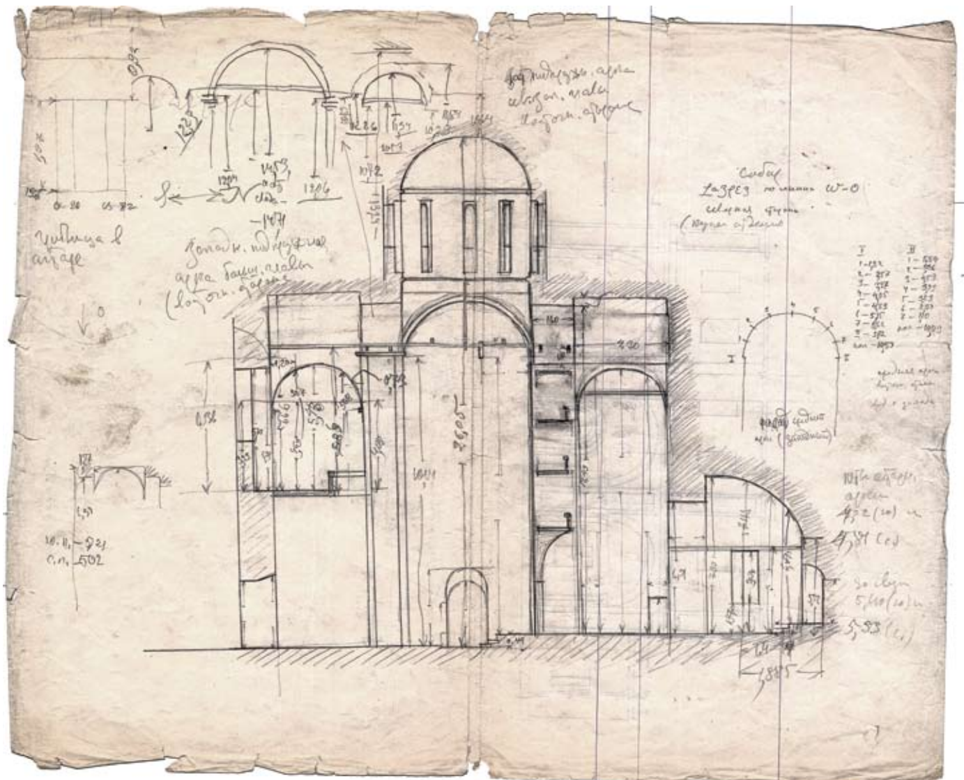
Вознесенский собор Вознесенского монастыря. Продольный разрез
