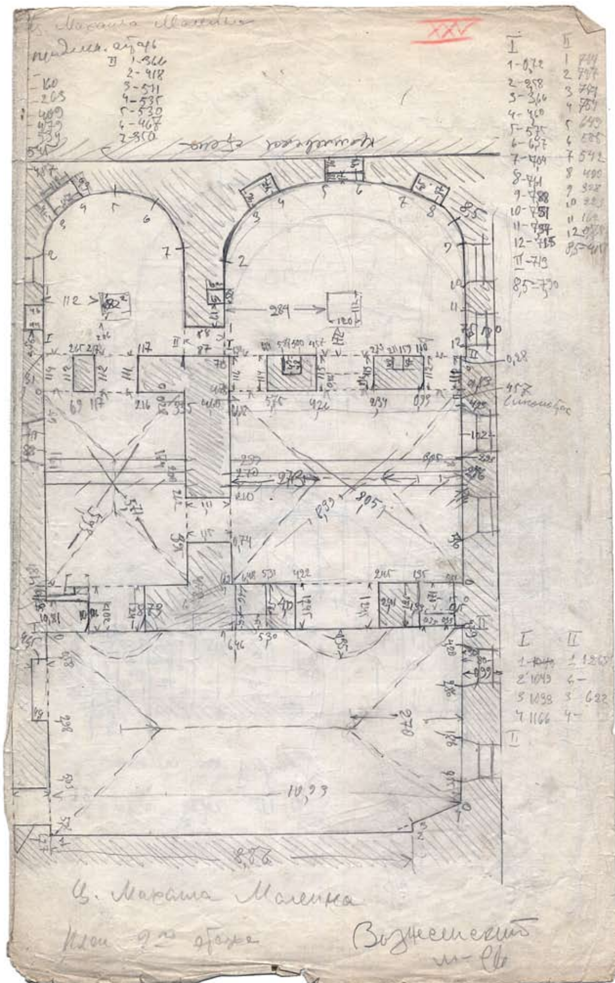
Церковь преподобного Михаила Маленка Вознесенского монастыря. План второго яруса
